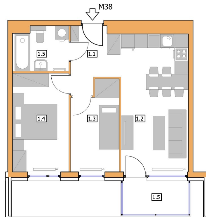
RZUT 1:100
