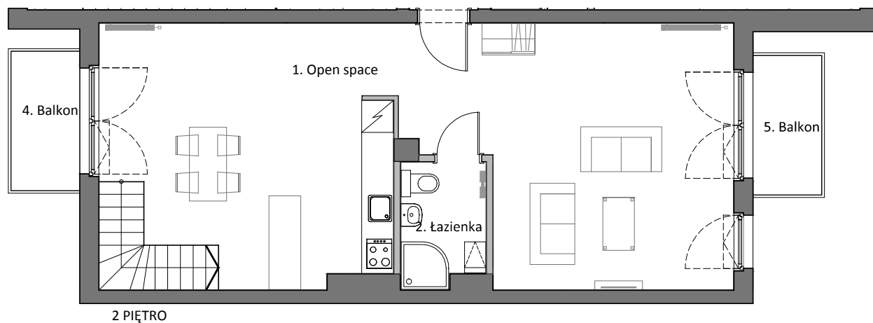
2 PIĘTRO
