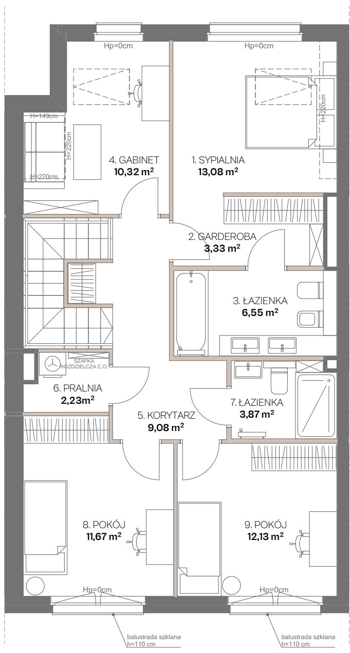
RZUT 1. PIĘTRA
