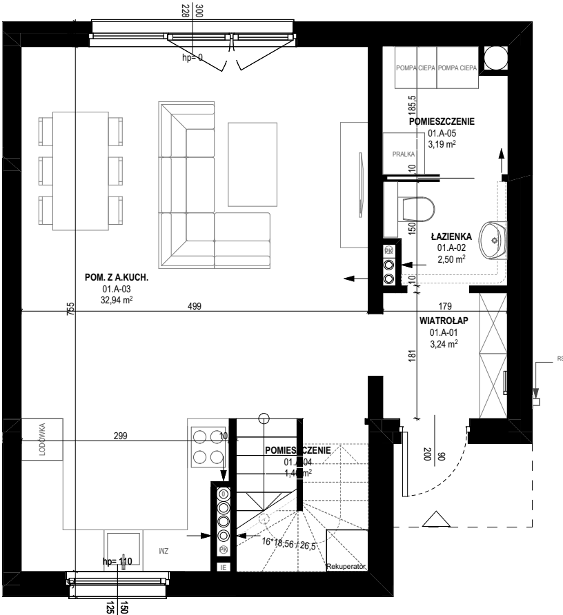
RZUT PARTERU
