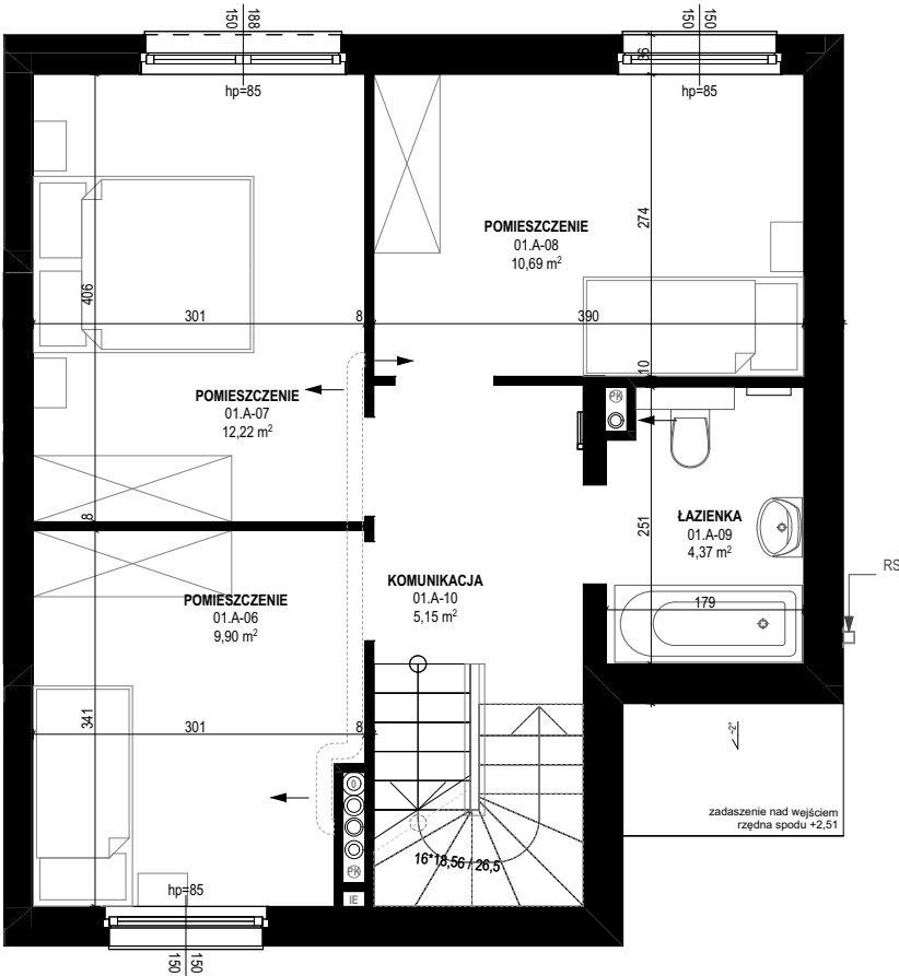
RZUT 1 PIĘTRA
