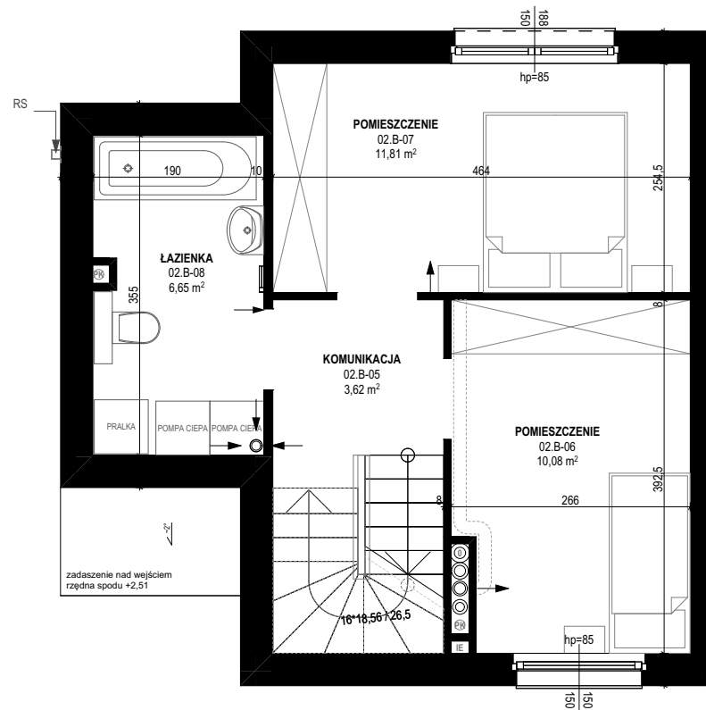
RZUT 2 PIĘTRA
