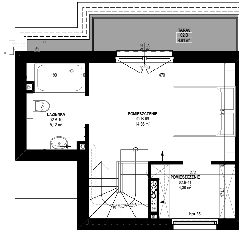
RZUT 2 PIĘTRA
