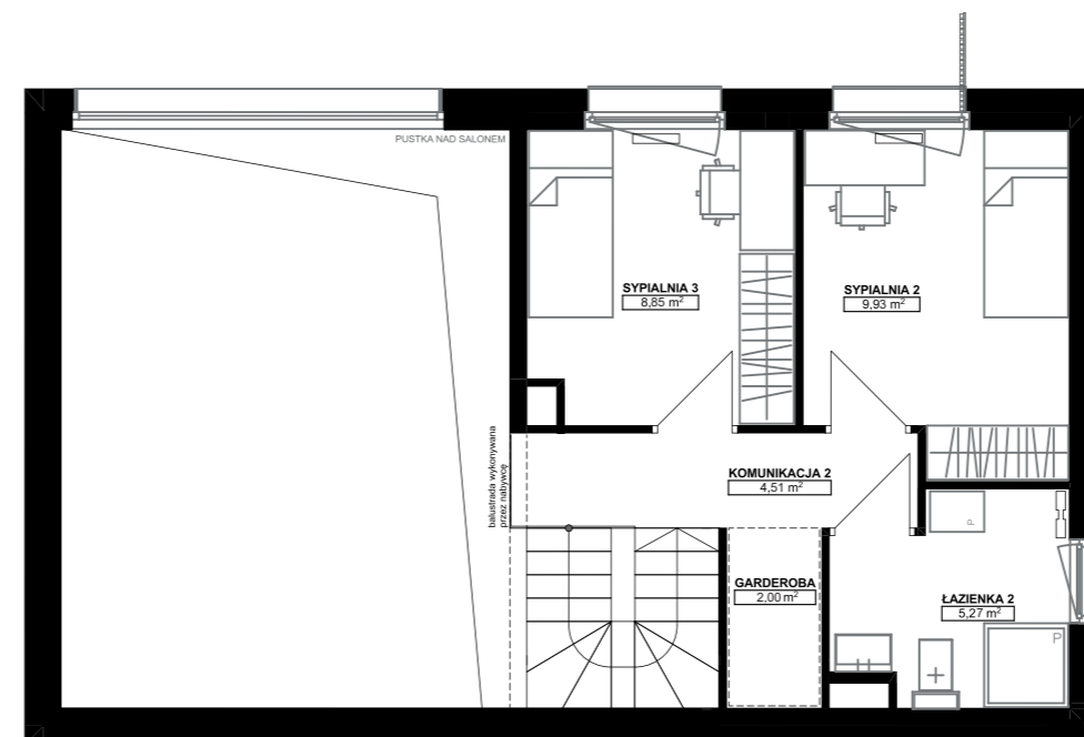
PIĘTRO I
