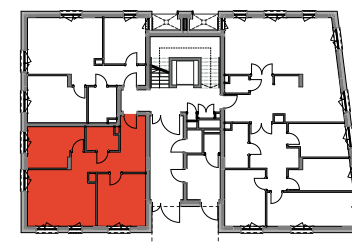
Schemat kondygnacji
