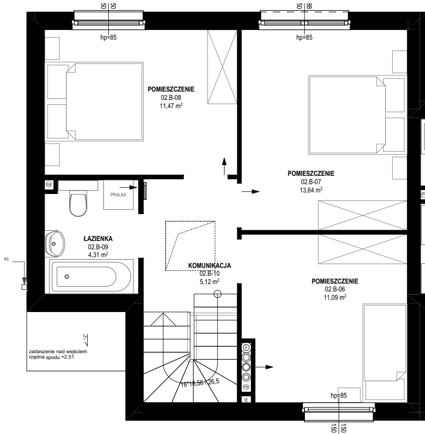
RZUT 1 PIĘTRA
