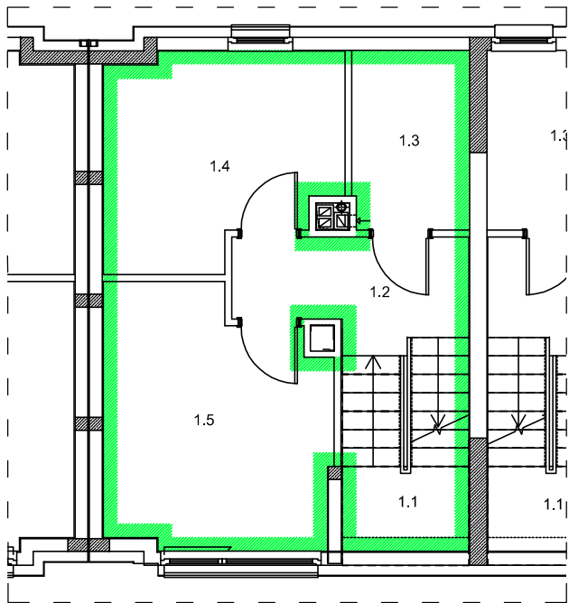
RZUT PIĘTRA I-GO BUDYNKU NR 11F LOKAL MIESZKALNY NR 2
