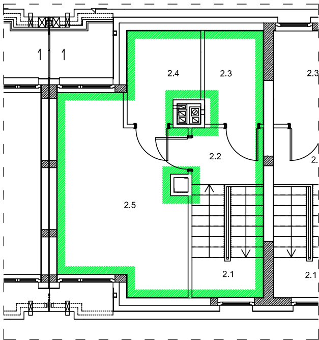
RZUT PIĘTRA II-GO BUDYNKU NR 11F LOKAL MIESZKALNY NR 2
