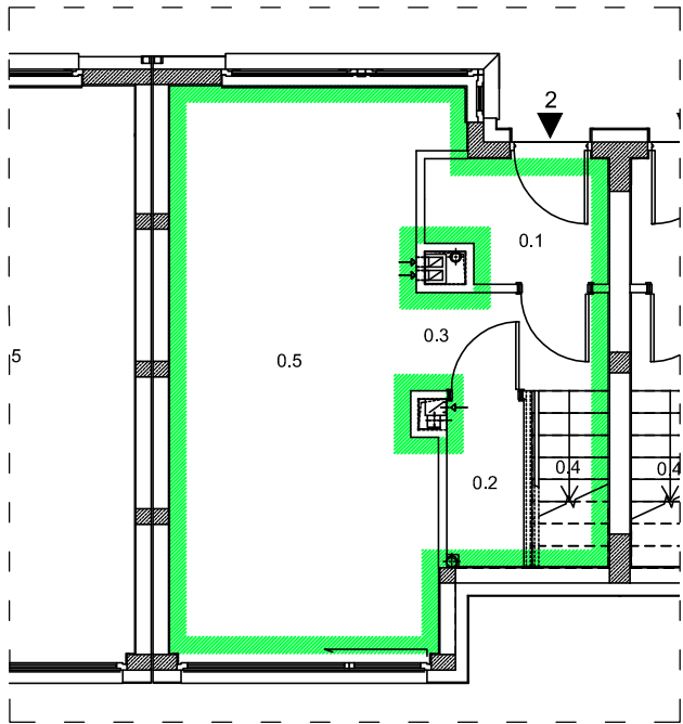
RZUT PARTERU BUDYNKU NR 11F LOKAL MIESZKALNY NR 2
