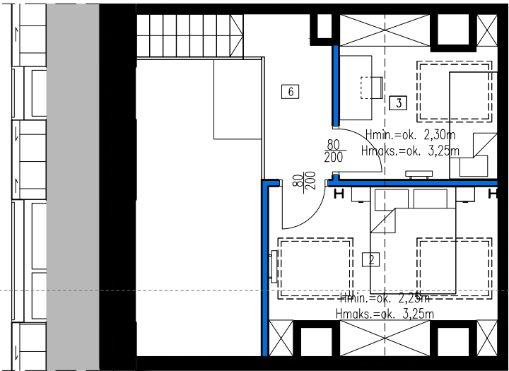
POZIOM + I
