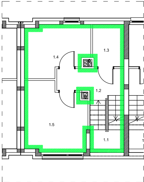
RZUT PIĘTRA I-GO BUDYNKU NR 11H LOKAL MIESZKALNY NR 2
