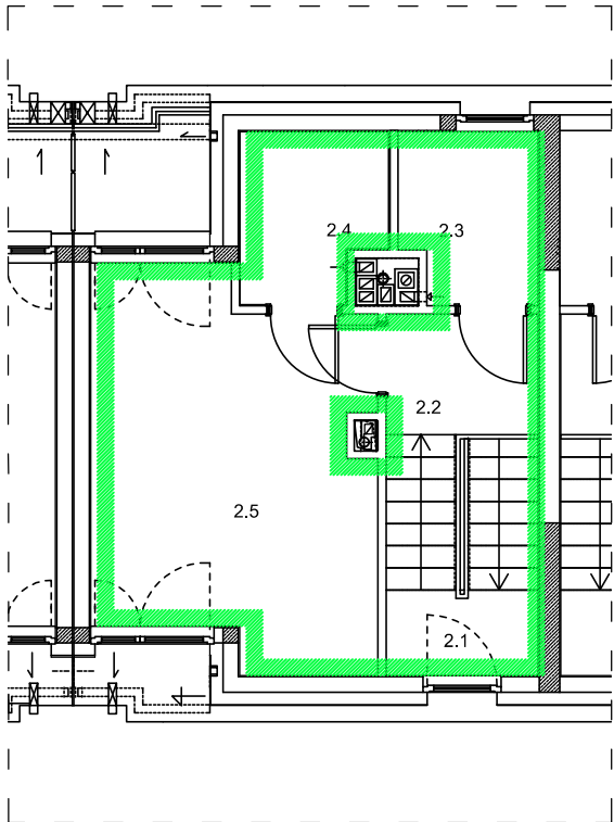
RZUT PIĘTRA II-GO BUDYNKU NR 11H LOKAL MIESZKALNY NR 2
