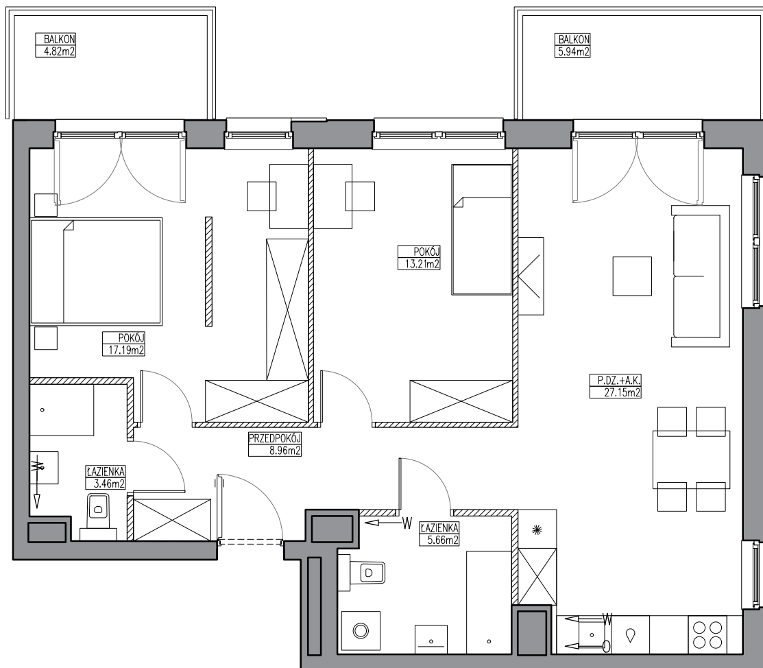
SCHEMAT LOKALU MIESZKALNEGO NA 1 PIĘTRZE
