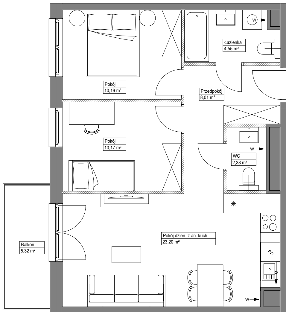
SCHEMAT LOKALU MIESZKALNEGO NA PIĘTRZE
