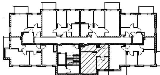
Zestawienie pomieszczeń - BM13
