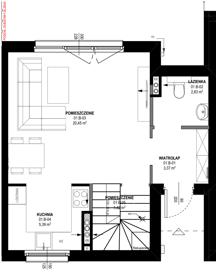
RZUT 1 PIĘTRA
