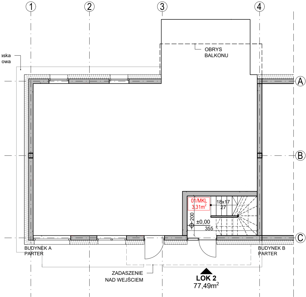
RZUT PARTERU
