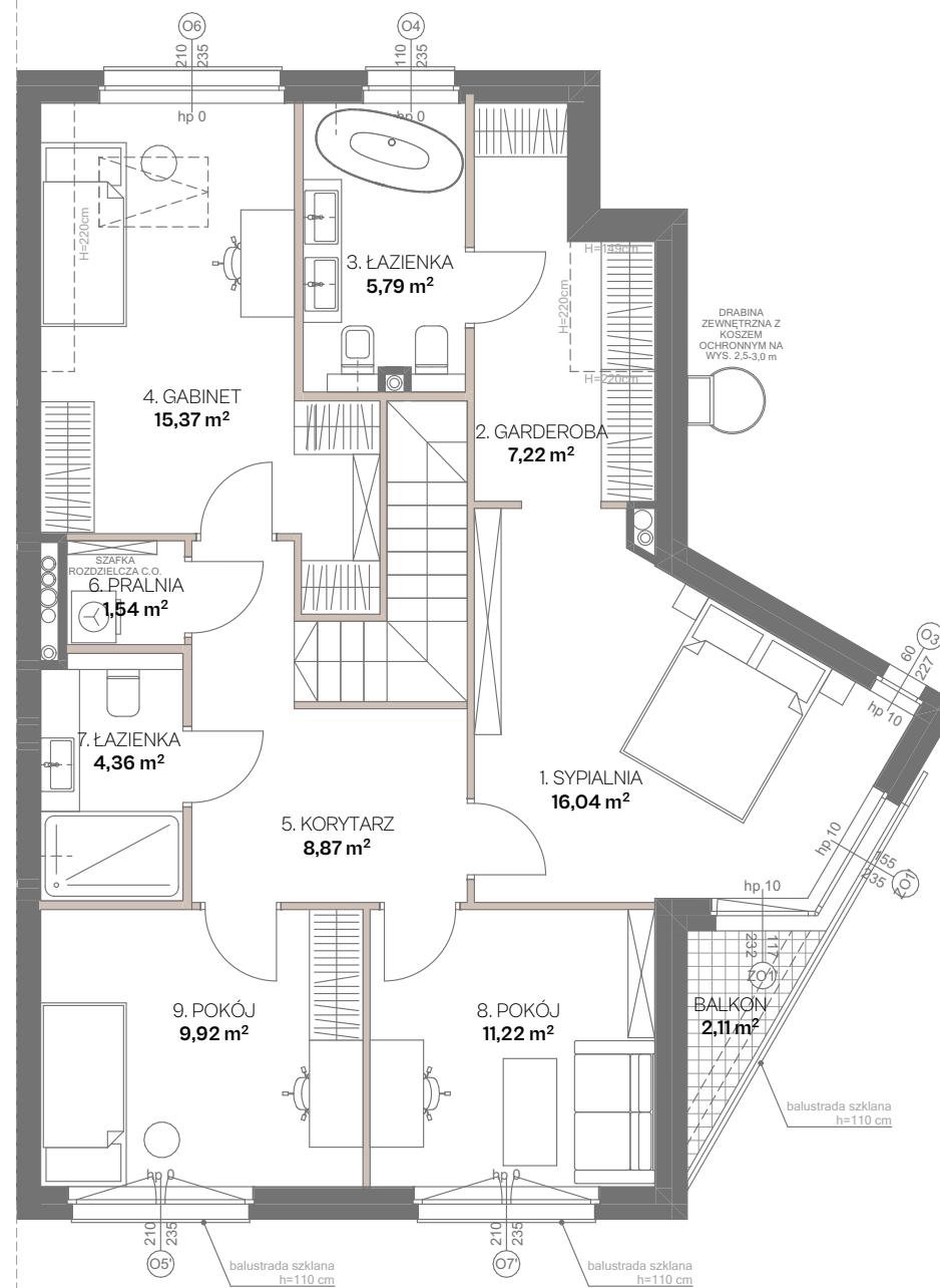
RZUT 1. PIĘTRA
