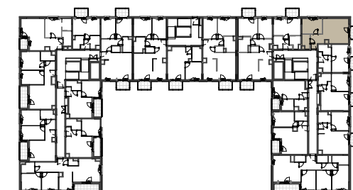
Rzut piętra 2
