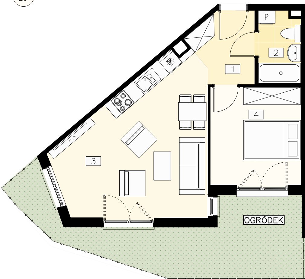
RZUT KONDYGNACJI
