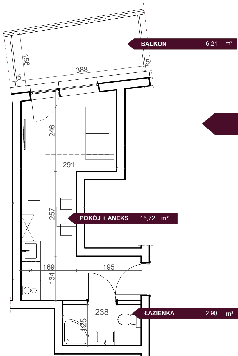
L.A.1.9 - I PIĘTRO
