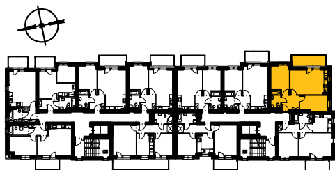
RZUT III PIĘTRA
