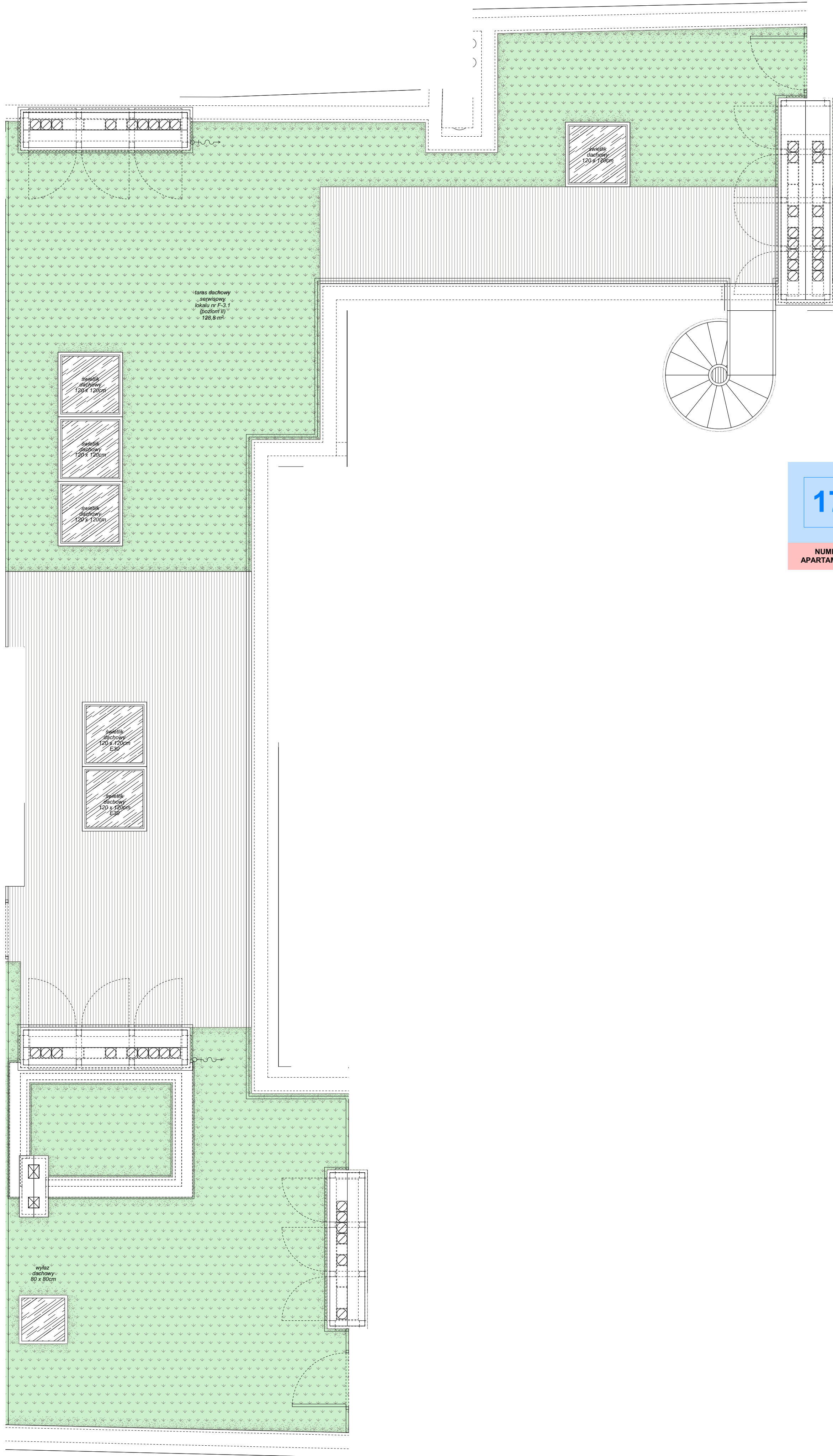
RZUT TARASU DACHOWEGO skala 1:50
