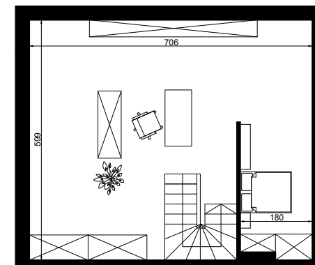
Rzut poddasza
