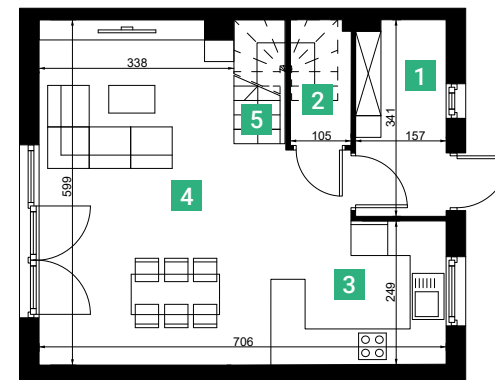
Rzut parteru
