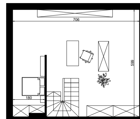
Rzut poddasza
