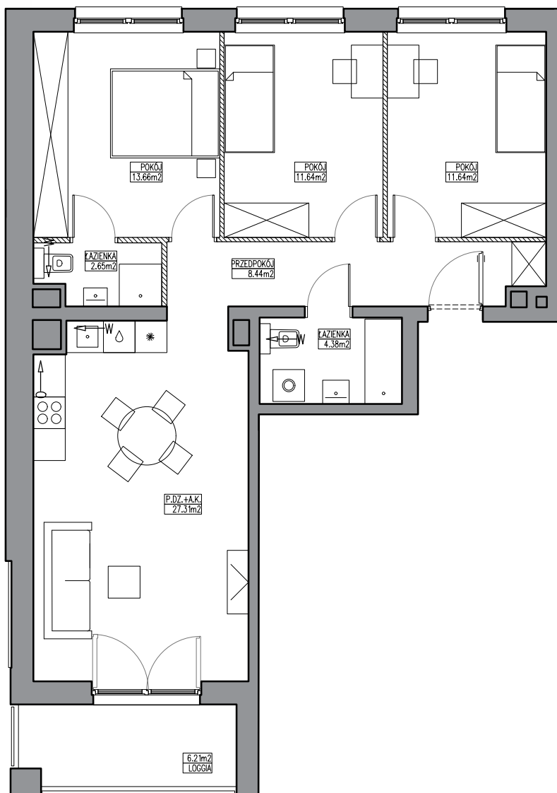
SCHEMAT LOKALU MIESZKALNEGO NA 1 PIĘTRZE
