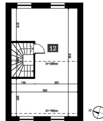
Rzut poddasza
