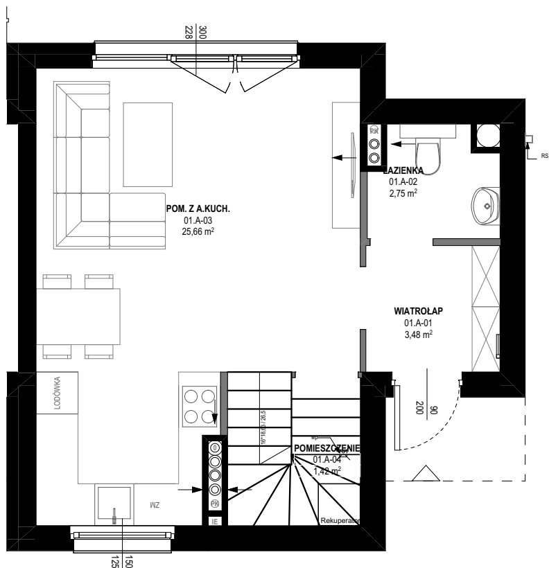
RZUT PARTERU
