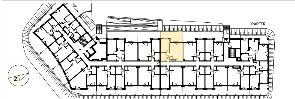
RZUT KONDYGNACJI
