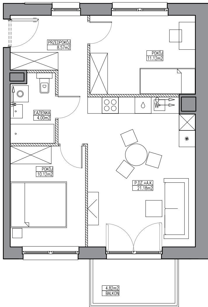
SCHEMAT LOKALU MIESZKALNEGO NA 4 PIĘTRZE
