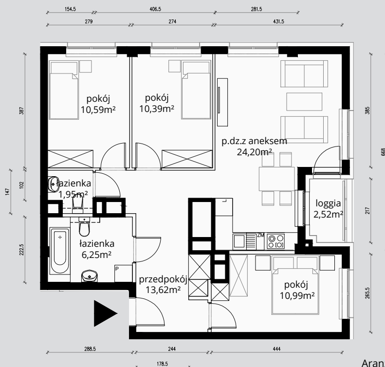
RZUT KONDYGNACJI 16 PIĘTRO
