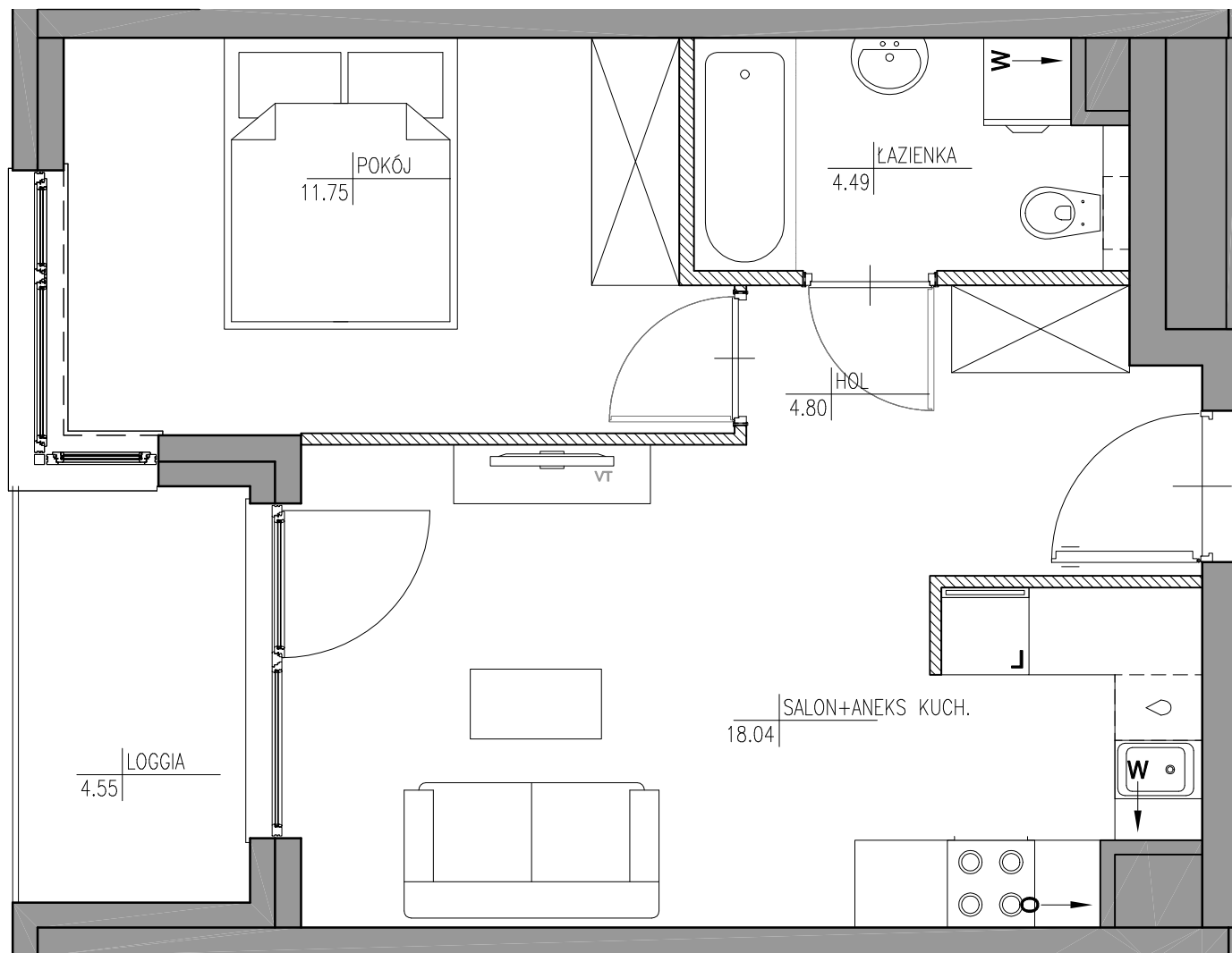
SCHEMAT LOKALU MIESZKALNEGO NA PIĘTRZE
