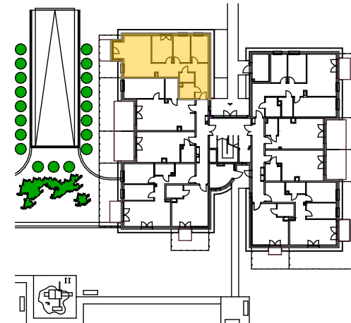
BUDYNEK 2 - PARTER
