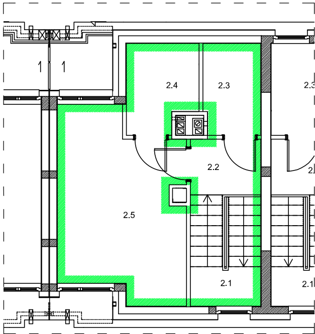
RZUT PIĘTRA II-GO BUDYNKU NR 9G LOKAL MIESZKALNY NR 1
