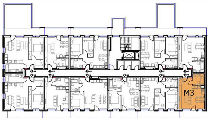
BUDYNEK B - 1 PIĘTRO
