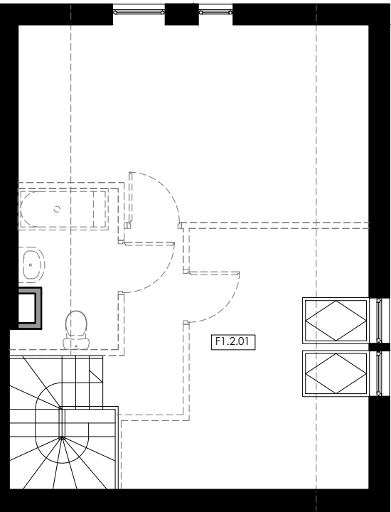
PODDASZE
