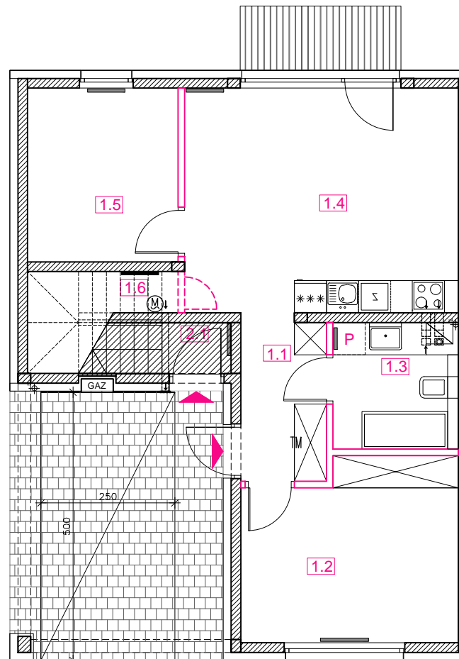
RZUT PARTERU
