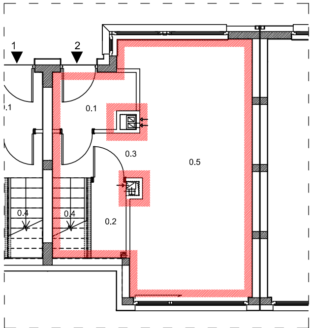
RZUT PARTERU BUDYNKU NR 9K LOKAL MIESZKALNY NR 2
