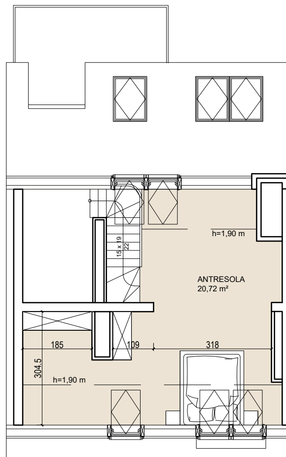
Poziom 2 (antresola)
