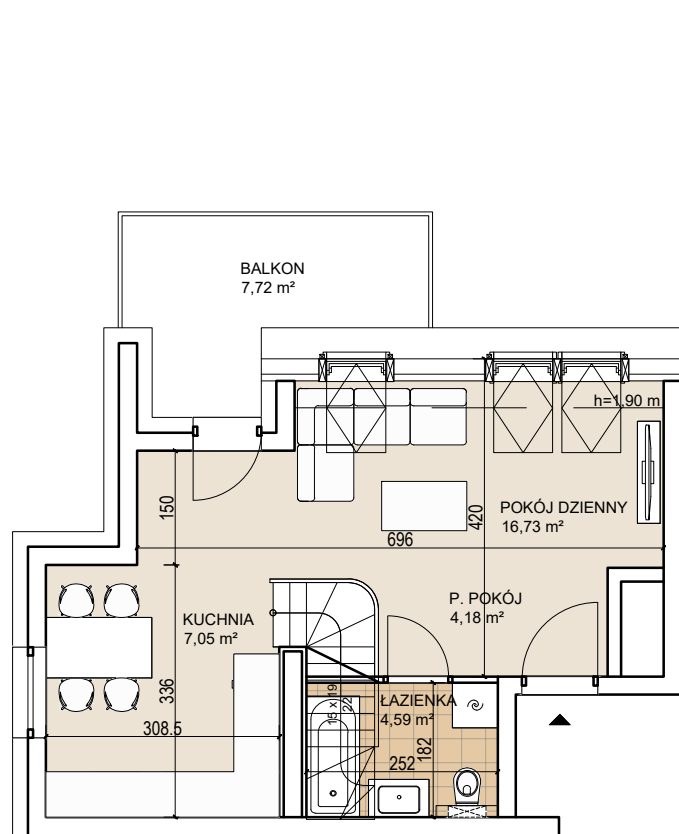
Poziom 1
