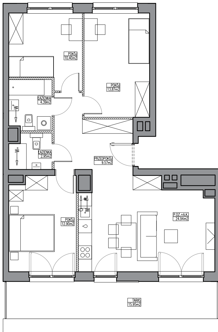
SCHEMAT LOKALU MIESZKALNEGO NA 7 PIĘTRZE
