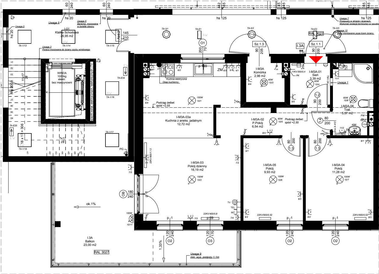
RZUT w skali 1:100
