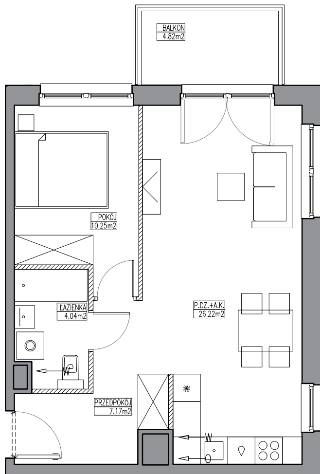
SCHEMAT LOKALU MIESZKALNEGO NA 4 PIĘTRZE
