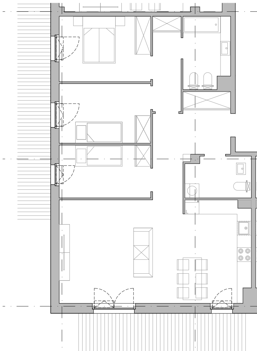
ZESTAWIENIE POWIERZCHNI - MIESZKANIE M-4P, POZIOM +11
