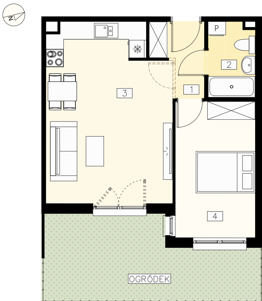
RZUT LOKALU
