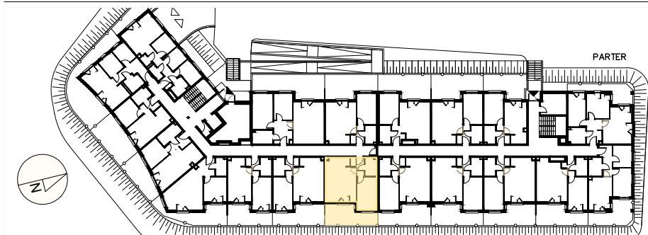
RZUT KONDYGNACJI
