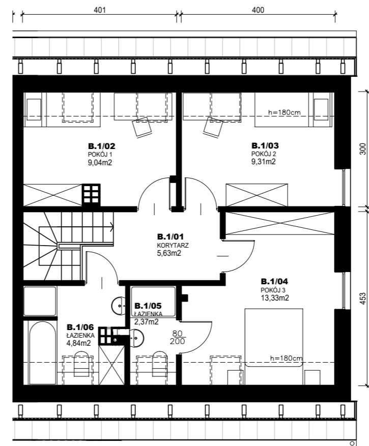
RZUT PODDASZA
