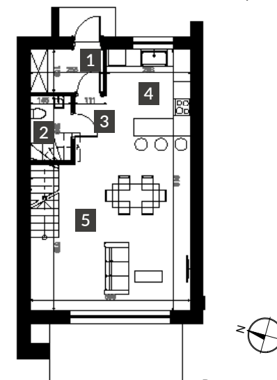
Rzut parteru
