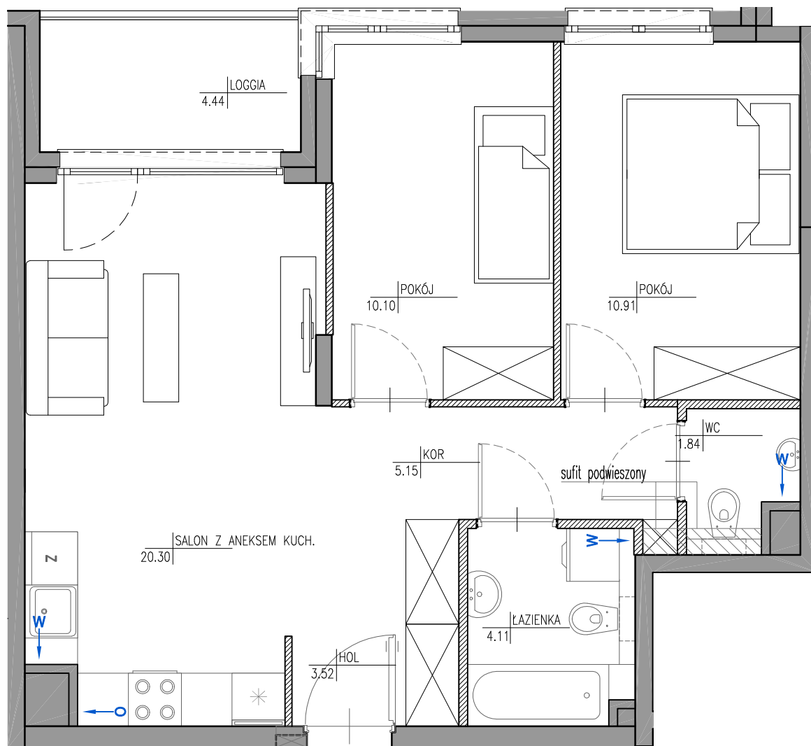
SCHEMAT LOKALU MIESZKALNEGO NA RZUCIE
