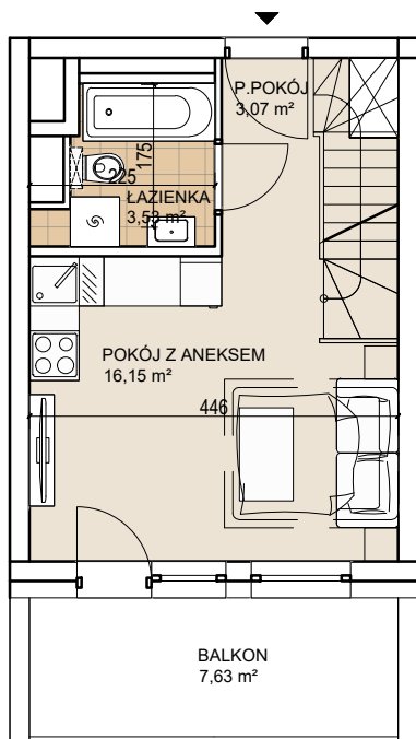
Poziom 1
