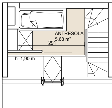
Poziom 2 (antresola)
