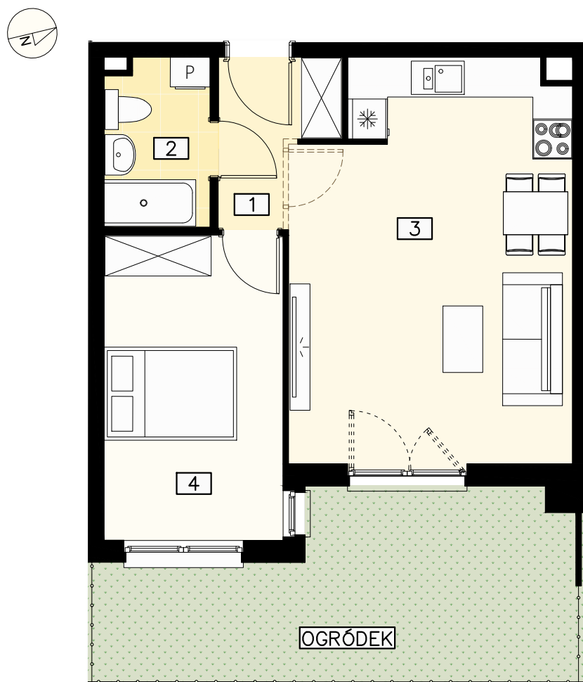
RZUT LOKALU
