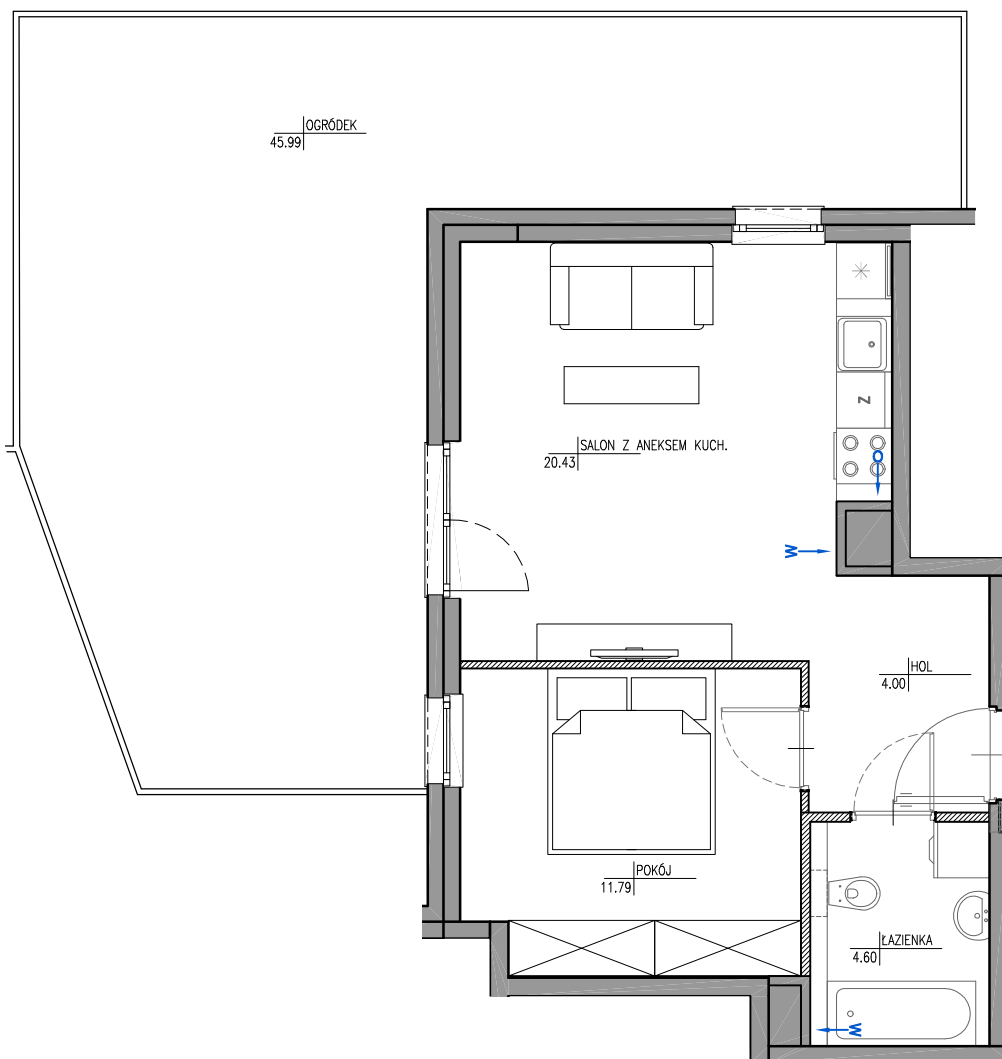
SCHEMAT LOKALU MIESZKALNEGO NA RZUCIE
