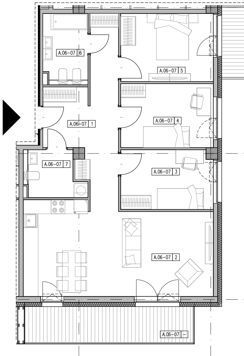
ZESTAWIENIE POWIERZCHNI - MIESZKANIE M-3P, POZIOM +6
